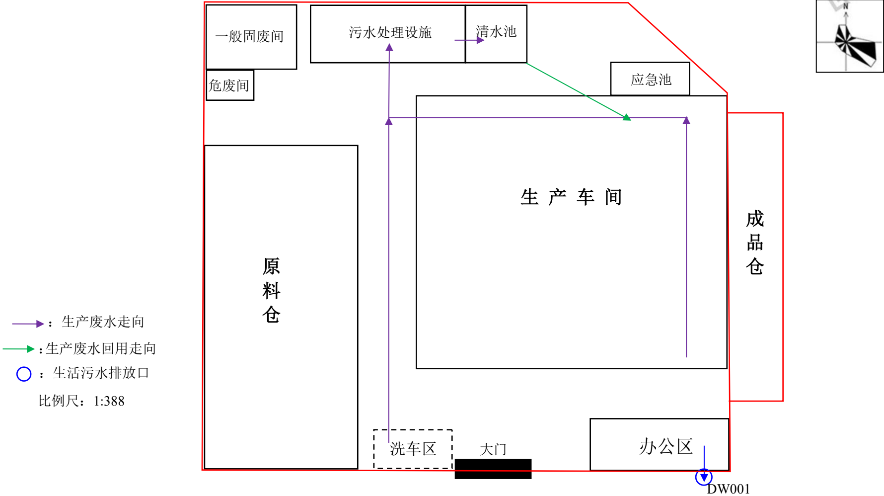
附图 5 项目总平面布置示意图
