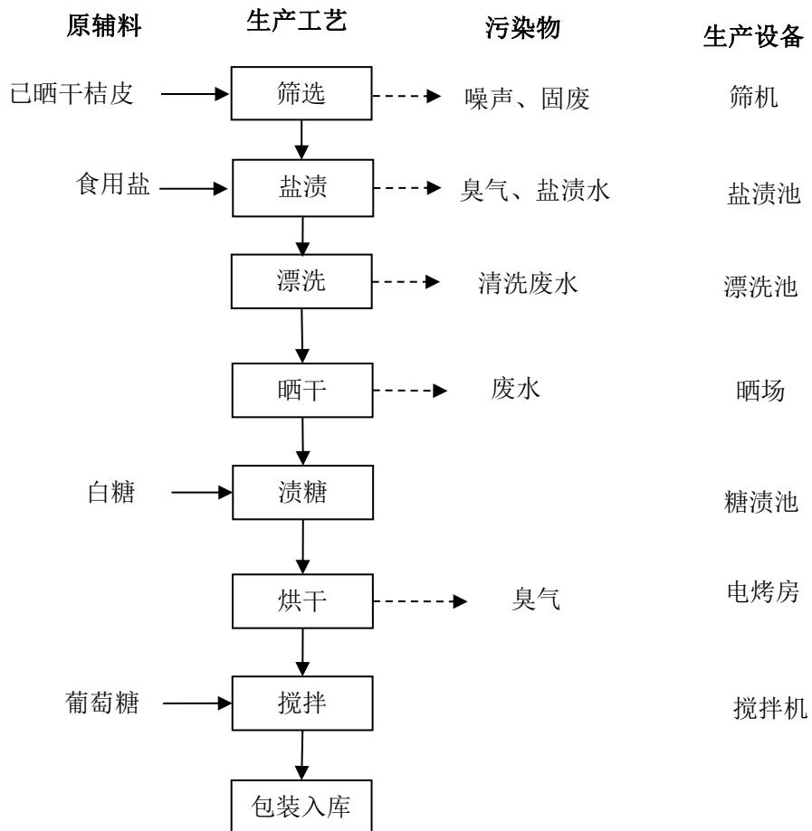
图 2-1 陈皮加工工艺流程及产污环节
