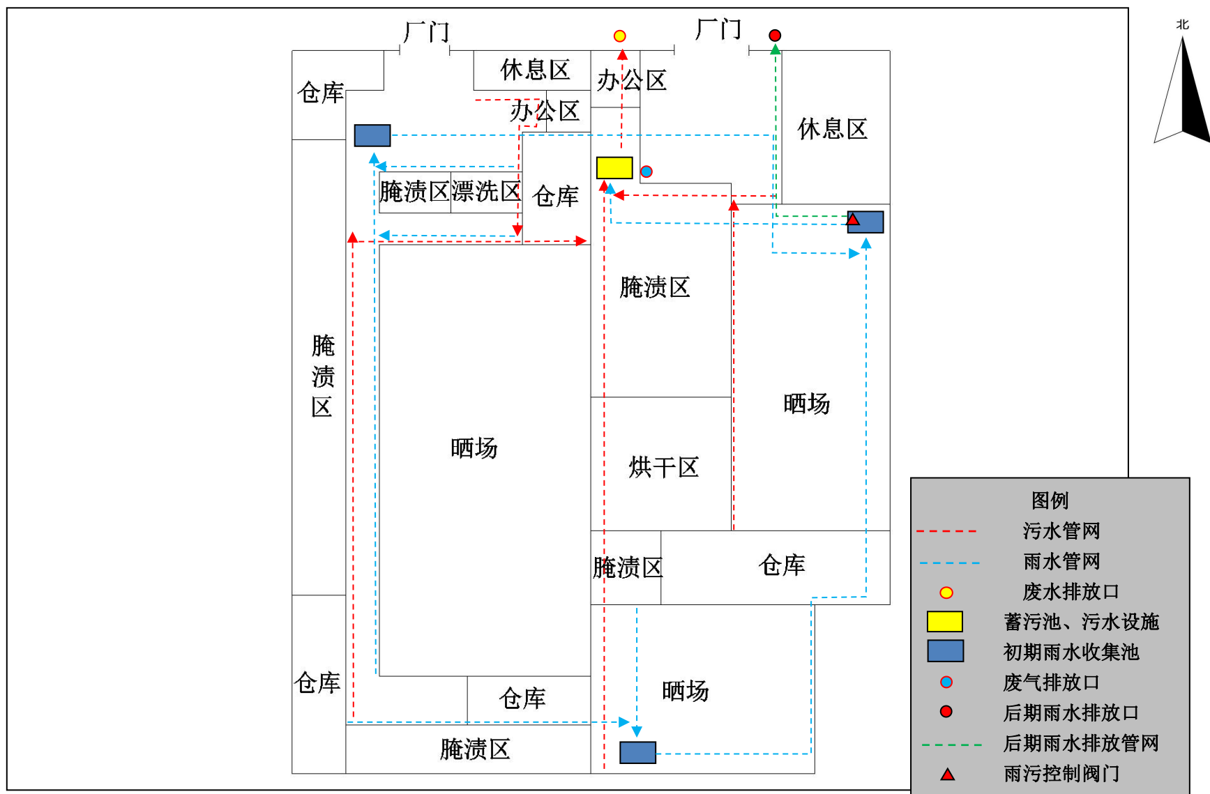
附图 5 本项目平面布置图
